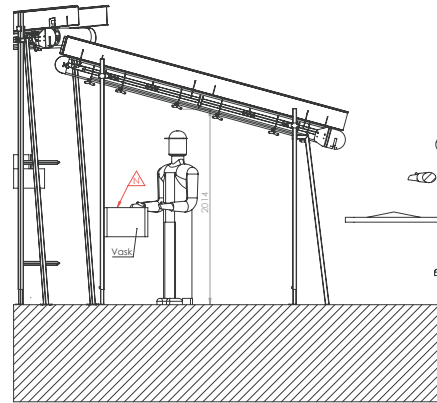
SECTION D-D SCALE 1 : 20
