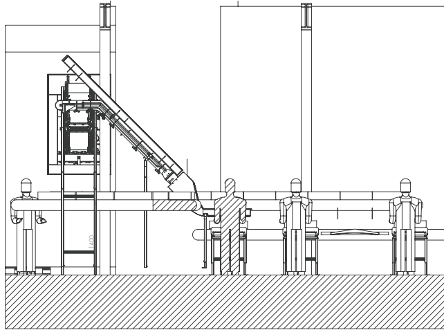
SECTION a-b SCALE 1 : 25
