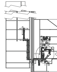
SECTION A-A SCALE 1 : 20
